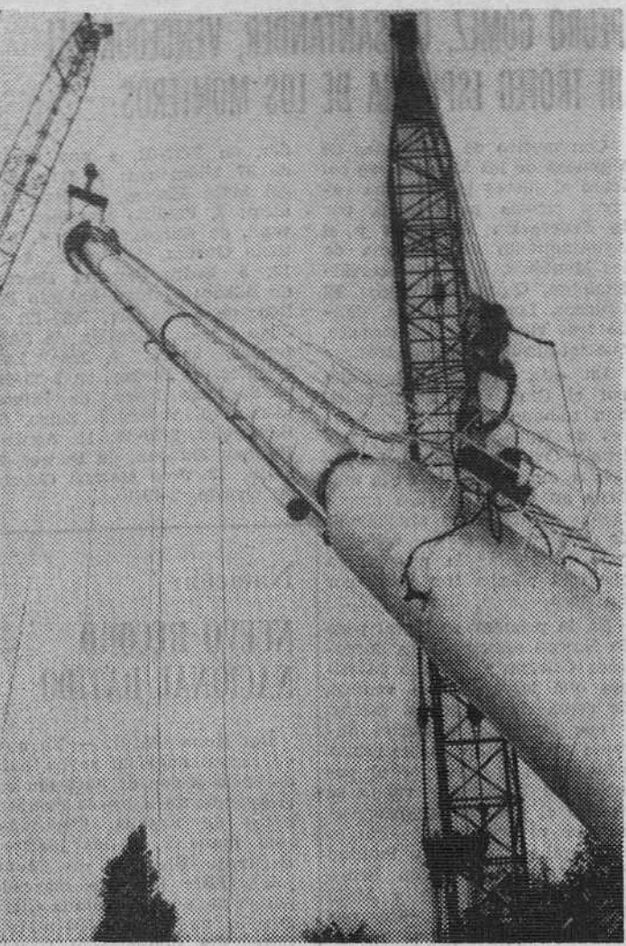
Apuntando hacia el cielo como si se tratara de un potente cañón o un gran telescopio el fotógrafo ha captado esta imagen de una chimenea de 46 metros de altura para una factoría cuando es elevada con dos grúas para ser instalada. La foto, en Hamburgo (Alemania). — (Foto FIEL)
