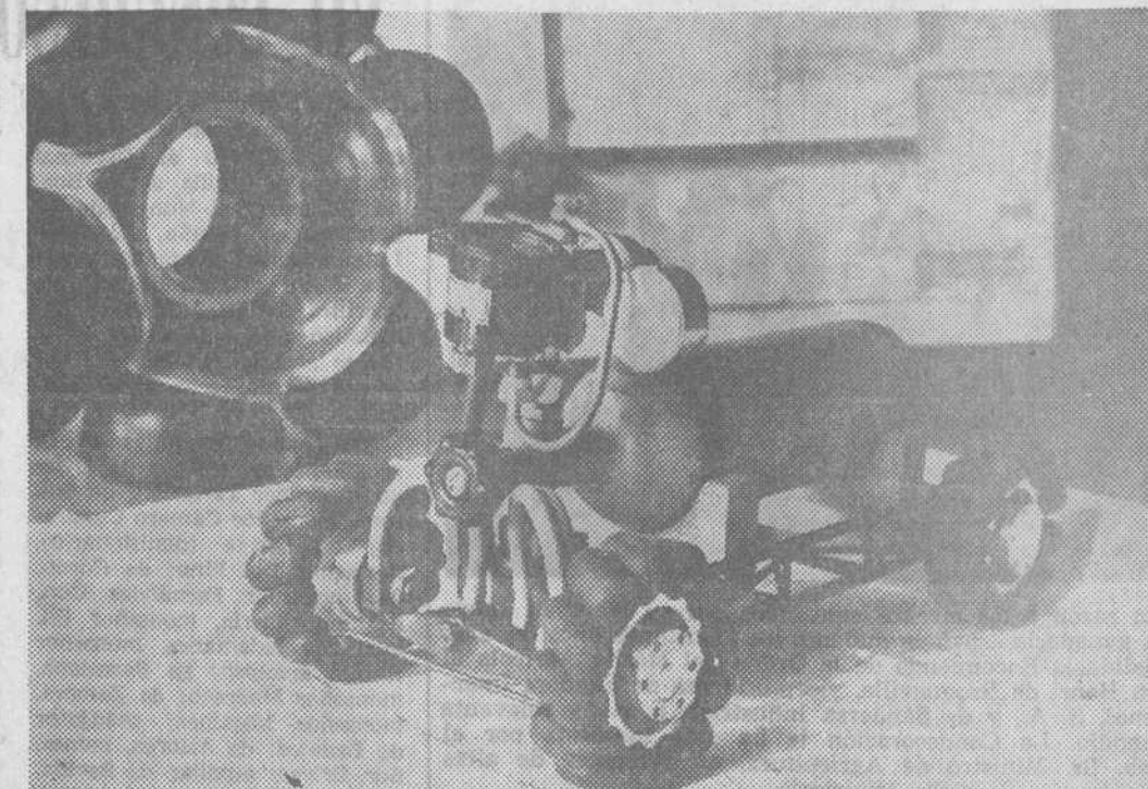
El primer prototipo del "Rotoped", vehículo con un nuevo y revolucionario tipo de fuerza impulsora, está siendo construido en el Instituto de Investigaciones de Vehículos de Motor, en Praga. El señor Julius Mackerle es el inventor, consistente en una especie de doce bolas fijadas en la periferia de cada rueda que por aire comprimido logran el movimiento y la fuerza impulsora. En efecto, el aire a presión, mediante un distribuidor en la propia rueda, pasa de una bola a otra, concretamente de la rueda. Diversas firmas de los Estados Unidos especializadas en investigaciones espaciales y fabricación de equipos se han interesado por este revolucionario sistema. — (Foto FIEL).
