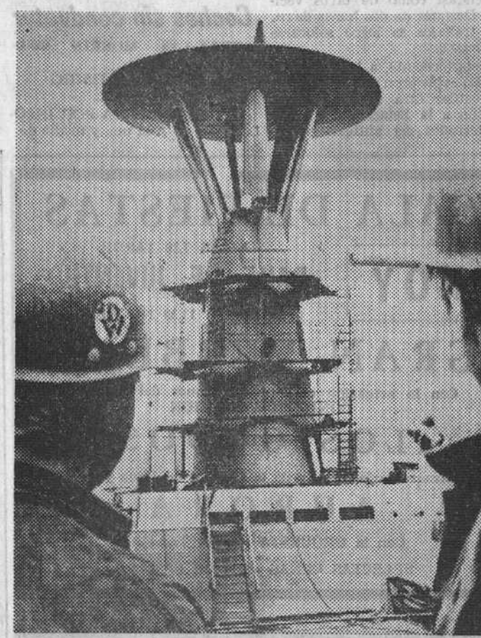
El más moderno barco alemán, que se está construyendo en los astilleros Werft de Hamburgo, llevará esta curiosa chimenea sin precedentes en la historia de la navegación marina. Los diseñadores están orgullosos de su obra que, a pesar de todo, no tiene una forma caprichosa. Se trata de un nuevo tipo de chimenea para que los pasajeros de cubierta no sean molestados por el humo y el hollín. Ocho meses de experimento han tardado en el Instituto Técnico de Berlín para dar con el diseño deseado, que tiene forma de mesa. — (Foto FIEL)
