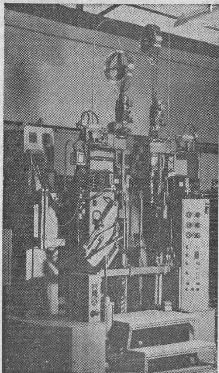
Máquina "Soudronic" de control electrónico para soldadura de elementos en atmósfera de gas inerte.
