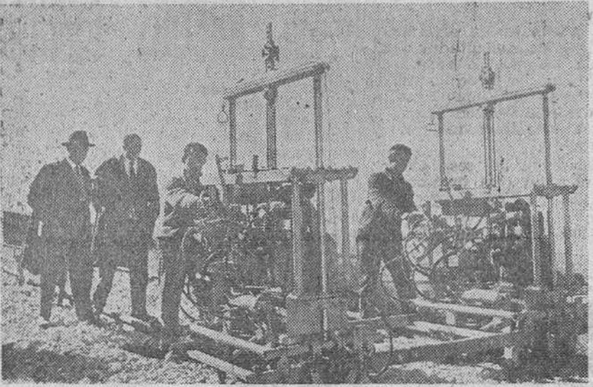
EMBRIDAD DE LA PAREJA RECIENTE COLOCADA EN LA VIA (Foto FEDE)
