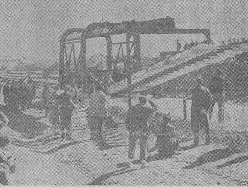
El director general de Ferrocarriles conversando con el gobernador civil acerca de determinadas características técnicas del Madrid-Burgos, en el trayecto visitado ayer. — Al pie, momento de la colocación de carriles en Villagonzalo Pedernales, como quien dice a la entrada de la ciudad.
