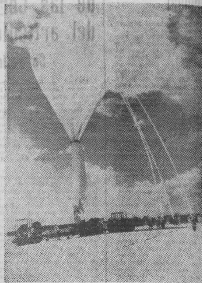
A través de tres tubos se bombea helio en el estratoscopio" hasta que alcanza un diámetro de 22 metros y medice. Uno de ellos ha llevado un telescopio de tres toneladas a 24.000 metros de altura. — (Foto Fiel)
