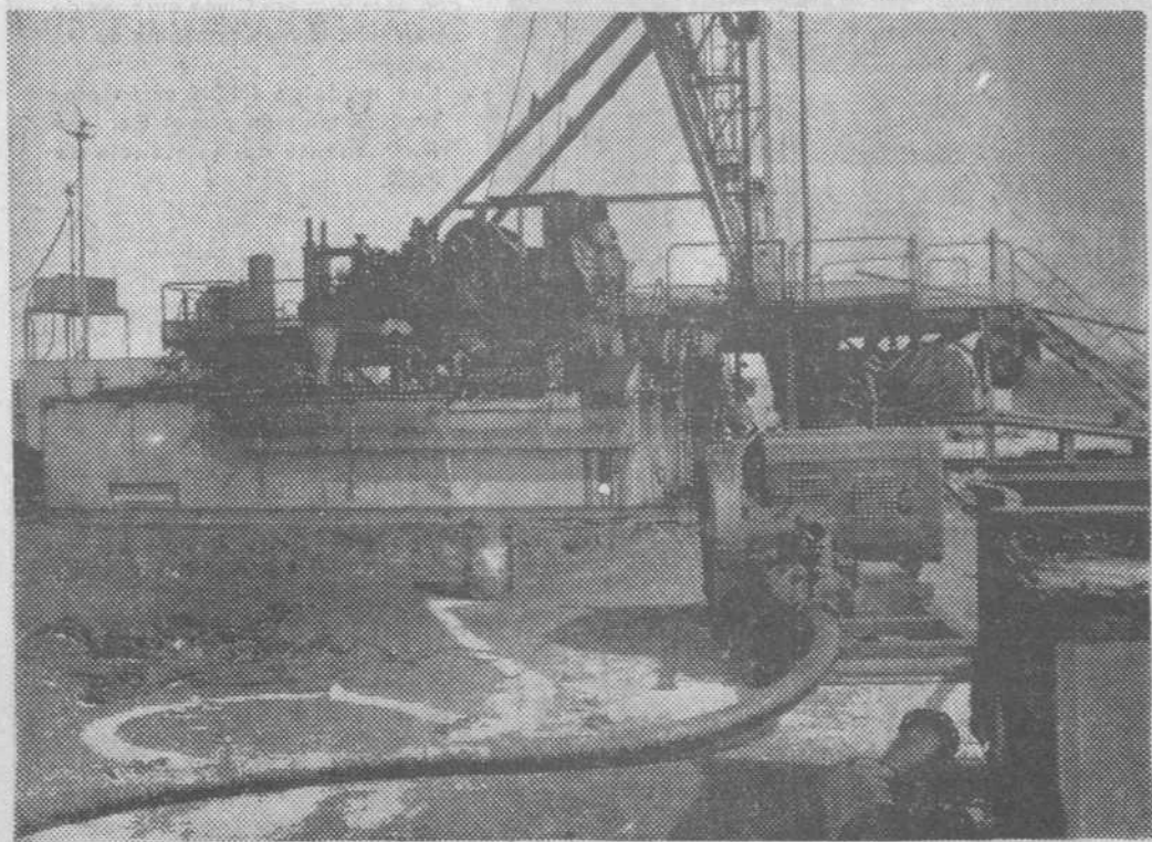
Aspecto que presentaba el "Ayoluengo 8" al finalizar la primera parte de las pruebas de producción industrial en el campo de la Lora. — (Foto Fede).
