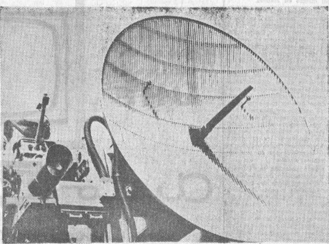
En Felixdorf (Austria) ha tenido lugar la presentación de nuevas armas para el Ejército austriaco, entre otras, este cañón anti-aéreo dirigido por radar. — (Foto Fiel)
