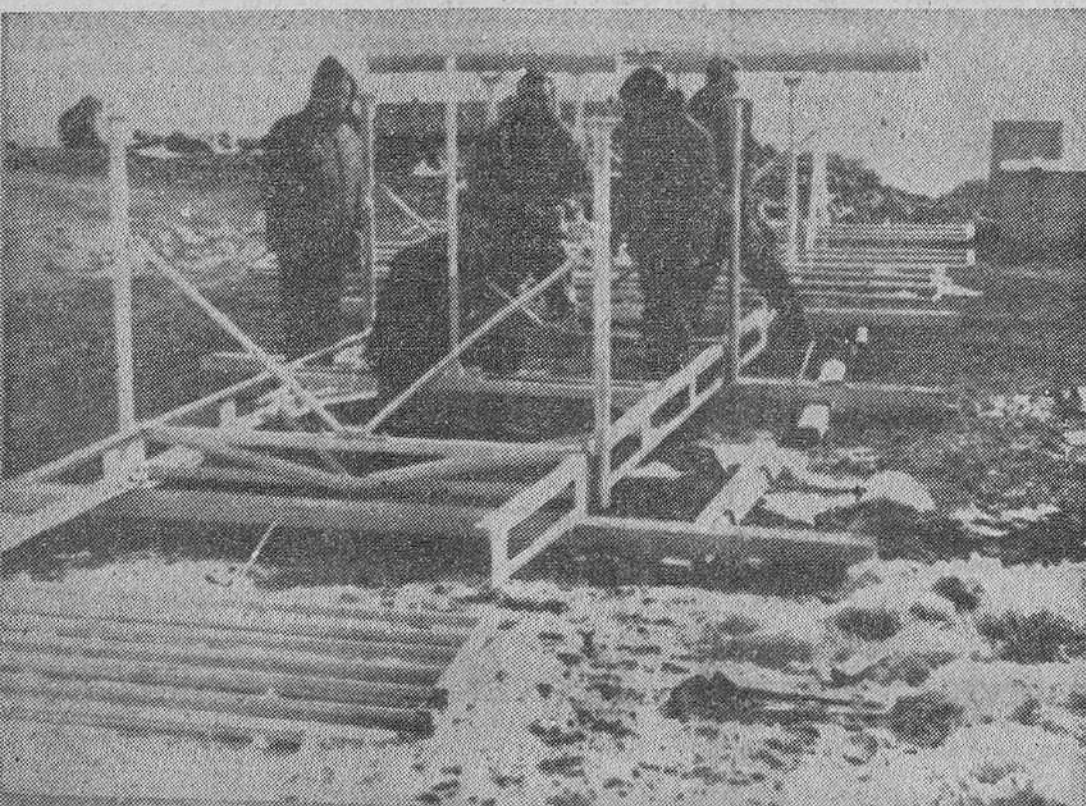
Las obras de montaje de la emisora de televisión de Izaña (Santa Cruz de Tenerife) han llegado a su fase final. En la foto el equipo de técnicos preparándose para izar la torre de la antena. (Foto «Fiel»)
