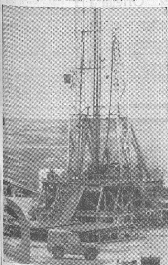
Estas imágenes fueron ayer captadas por «Fede» en el páramo de La Lora. En el grabado de la izquierda se reproduce un aspecto del tren de sonda en el «Ayoluengo número 2», mientras que la panorámica muestra la perspectiva general del tercer campamento petrolífero. La «foto» recoge el instante en que es izado el castillete del nuevo tren de perforación.
