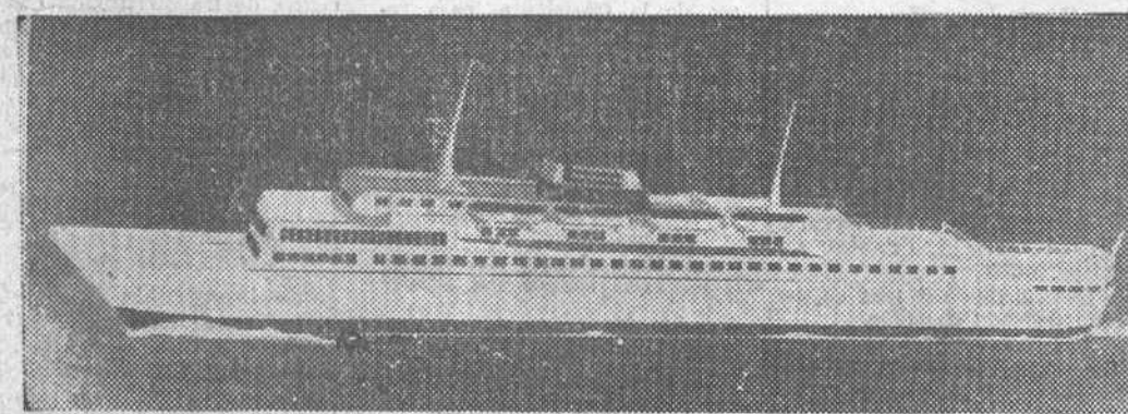
Un dibujo del primer mercante alemán construido después de la guerra y que será botado en 1966. Medirá 116 metros de eslora por 16 de manga. Desplazará 5.000 toneladas de registro bruto y tendrá una capacidad para 300 pasajeros, con un garaje en cubierta para 50 ó 60 automóviles. Contará además con piscina, baño sauna y cada cabina tendrá cuarto de baño propio. (Foto Fiel)
