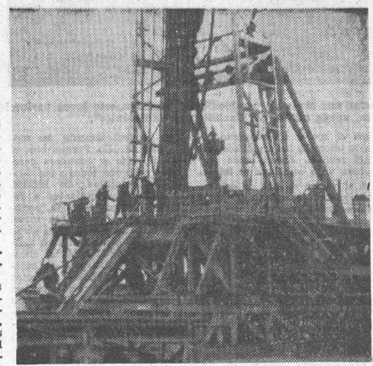
El personal del tren de sondeo del «Ayoluengo número 2» en plena acción de su trabajo, durante las maniobras con el largo varillaje de acero. (Foto FEDE)
