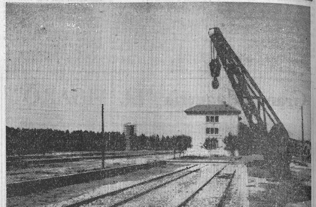
He aquí dos aspectos del estado actual de las obras del ferrocarril directo Madrid-Burgos, en el tramo Aranda-Burgos. En la parte superior, obreros trabajando en el montaje de los carriles. En segundo lugar, una vista de la estación del ferrocarril, en Aranda. (Fotos Roma).
