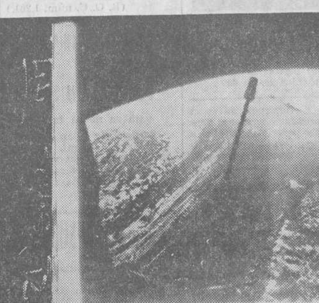
Centro espacial Houston. — Desde su altura record, los astronautas de la nave espacial «Geminis-11» consiguieron esta bella fotografía de nuestro planeta. — (Telefoto UPI-CIFRA)
