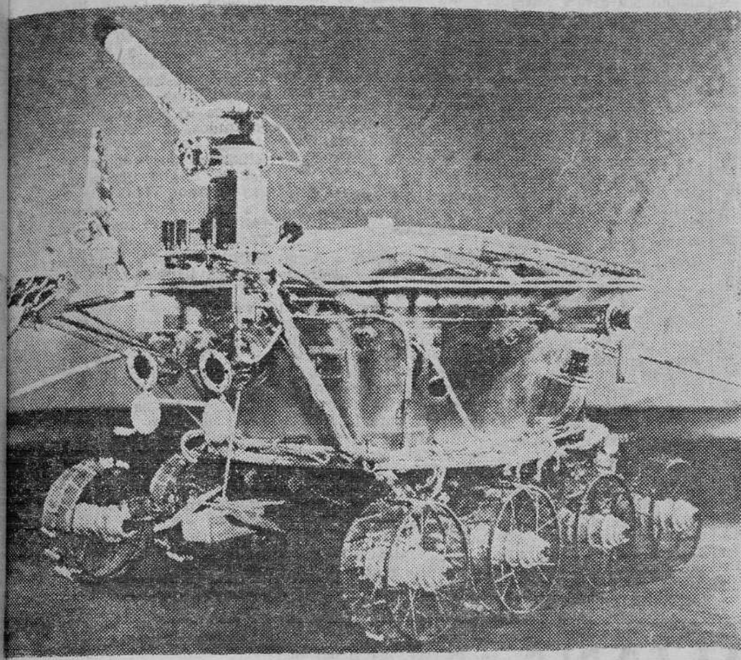
El «Lunojod I», vehículo automático y autopropulsado, ha explorado el suelo lunar, en el llamado Mar de las Lluvias, durante cerca de un año. — (Foto Efe)
