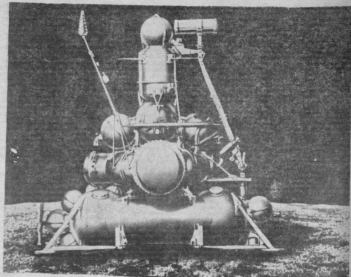
La nave espacial y laboratorio automático soviético «Luna 16». — (Foto Efe)
