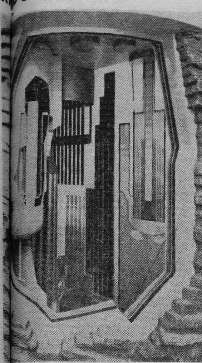
Este reactor rápido ha sido presentado por Gran Bretaña en la exposición la Paz, celebrada en Ginebra. Las características de este reactor construyendo en la ciudad escocesa de Dounreay, son: 2,1 metros de diámetro. El prototipo presentado en Ginebra presentaba un corte, con objeto de ilustrar al visitante sobre su funcionamiento. — (Foto Fiel)
