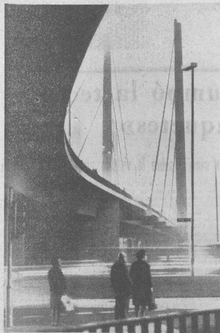
Tras cuatro años de construcción fue inaugurado recientemente el nuevo puente sobre el Rhin en Düsseldorf, que popularmente es conocido ya como el «puente del codo» por la curva que desarrolla sobre el río. Dos altos pilones de 115 metros soportan en la orilla izquierda el peso de la estructura. El puente tiene 564 metros de largo, de ellos 320 de carga libre sobre la corriente. Ha costado 170 millones de marcos. En esta foto le vemos iluminado al atardecer. — (Foto FIEL)
