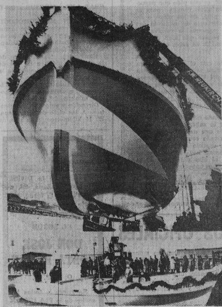
La primera embarcación de pesca construida en plástico en la República Federal de Alemania acaba de ser entregada en Bremerhaven a la naviera propietaria. Se trata de la lancha «Apolo», destinada para la pesca de quisquillas y gambas así como para la de bajura costera. La embarcación está construida con plátano reforzado con fibra de vidrio. Mide 16,30 metros de eslora, y 5 de manga, siendo su capacidad de carga de 30 toneladas. Se diferencia de las lanchas convencionales por su proa más marinera y su popa más ancha, lo que le asegura gran estabilidad. Todas las piezas de cubierta son también de plástico. Lleva un motor Diesel de 150 caballo, marítimos. Las fotos recogen un momento de su botadura. — (Foto Fiel)
