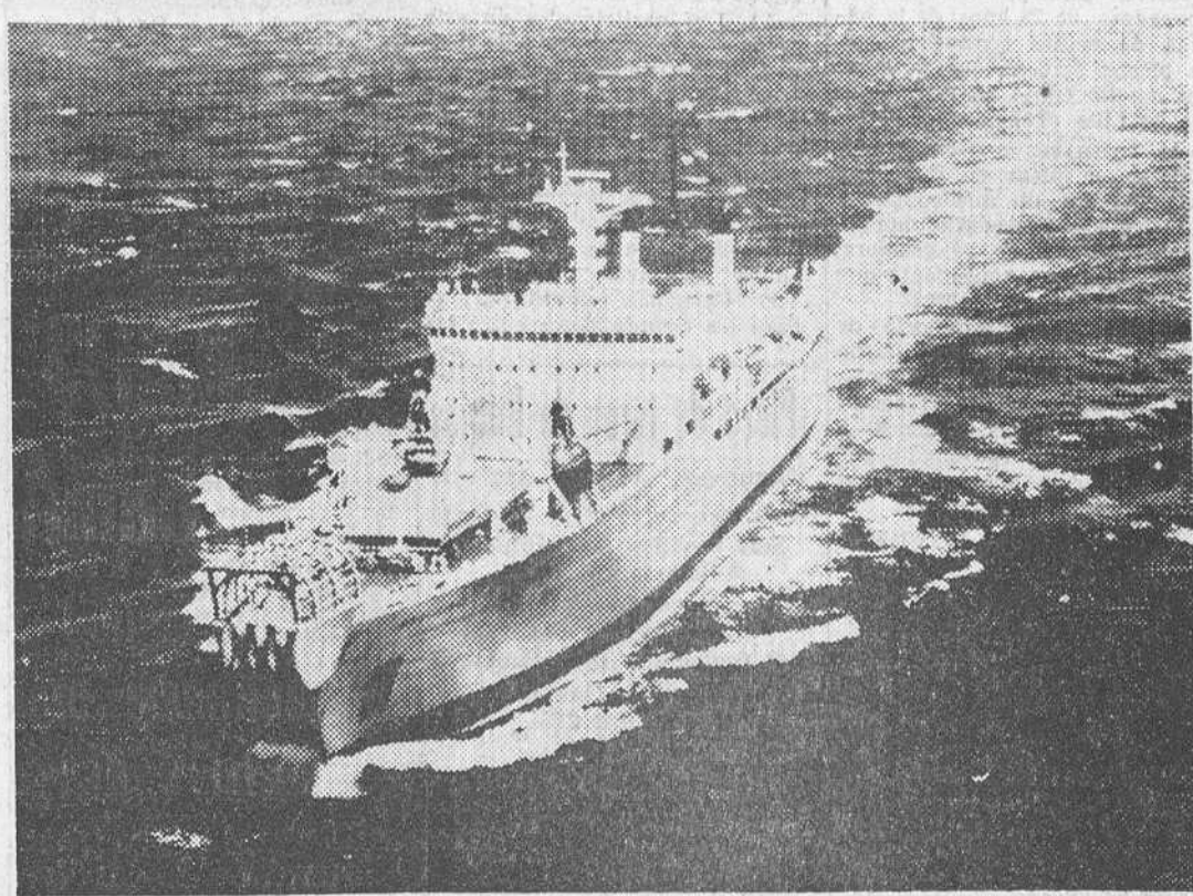
El barco norteamericano «Long Lines», especializado en la colocación de cables submarinos, ha sido el que ha llevado a cabo el tendido Nueva York-San Fernando-Roma. — (Foto EFE)
