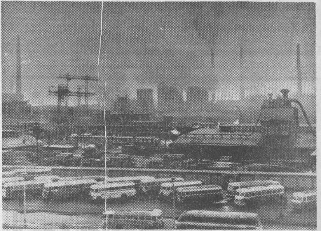
Los humos de las fábricas alemanas, como ésta de la cuenca de Ruhr, llegan hasta los bosques de Suecia, perjudicándolos. — (Foto Fiel)
