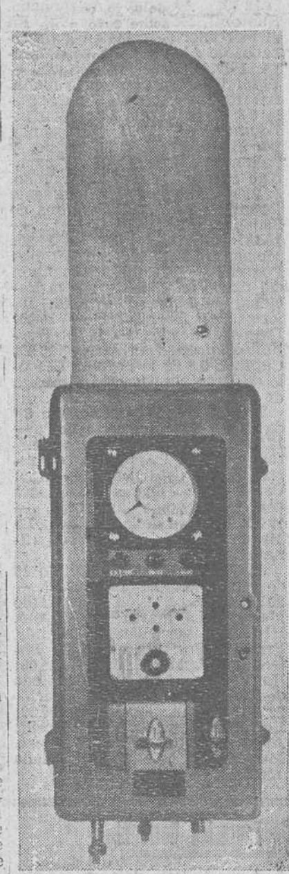
Un monitor para medir la actividad gamma, el T. P. A. Mark 1, para ser utilizado en las centrales nucleares y en sus proximidades.
