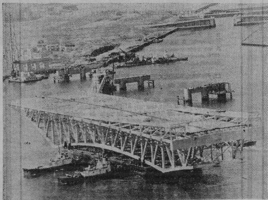
En el río Arakava, que desemboca en la Bahía de Tokio, se está construyendo un gigantesco puente. La foto nos muestra un tramo del puente que soportará el peso central. La estructura mide 195 metros de largo por cincuenta de ancho. Su peso es de unas 4.400 toneladas. Se tardaron cuatro horas en remolcar el tramo hasta la posición deseada. — (Foto FIEL)
