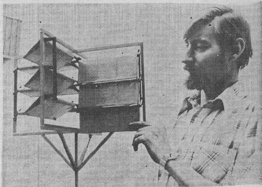
Esta construcción aparentemente tan sencilla que muestra aquí el inventor alemán Ernst Hohmann es una maqueta de su recién patentado «motor de viento» que, aprovechando la fuerza del viento, vía un tubo de aire comprimido, puede generar energía eléctrica a un precio muy reducido. — (Foto FIEL).
