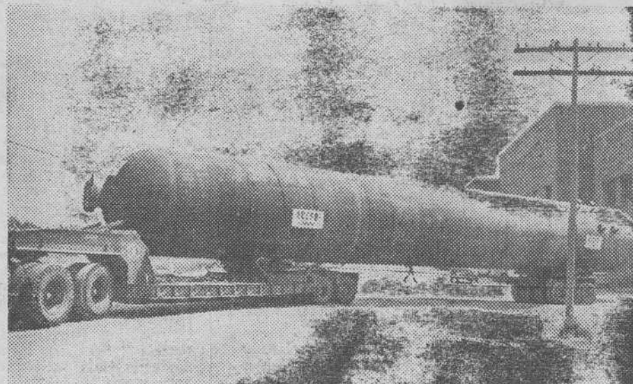
Este es el depósito gigante para la central nuclear de Vandellós (Tarragona) a su paso por la capital tarraconense. El depósito mide 30 metros de largo y de las dificultades de su transporte habla bien a las claras la fotografía. — (Foto "Fiel").
