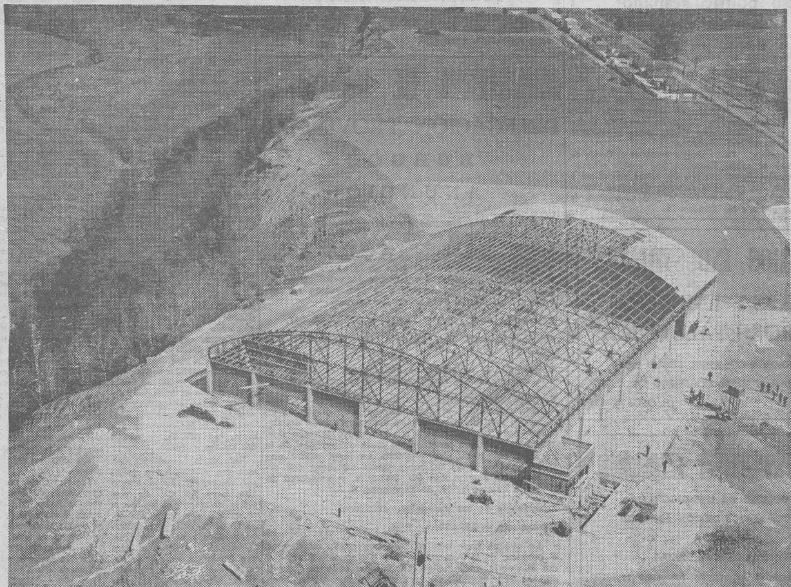
NAVE DE 50 M. DE LUZ, EN CARRION DE LOS CONDES (PALENCIA), CON CUBIERTA DE ESTRUCTURA METALICA, DISEÑADA Y CONSTRUIDA EN NUESTROS TALLERES.
