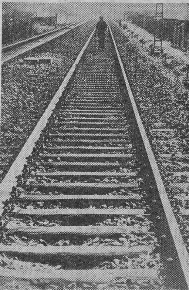
Un controlador recorre diariamente muchos kilómetros de vía en busca de posibles averías. Su trabajo no puede detectar defectos peligrosísimos que ahora quedaron de manifiesto gracias a la técnica de ultrasonidos. — (FOTO EFE-FIEL)
