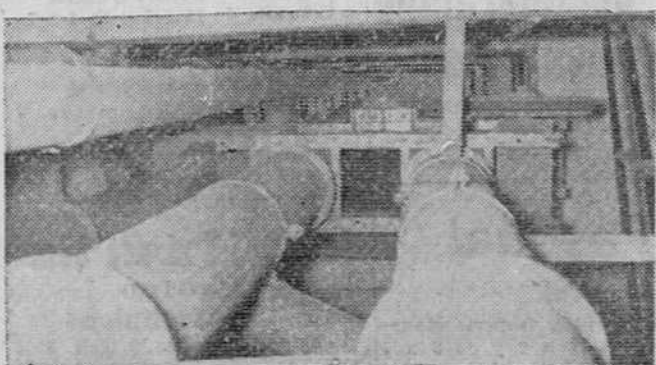
He aquí un detalle de la perfecta maquinaria con la que se realiza la limpieza y la elevación de materias primas, que posteriormente van pasando a las distintas secciones para su acabado
