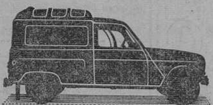
Renault-4 furgoneta Carga 350 kg. Altura útil 1,150 m. Volumen útil de carga 1,88 m³
