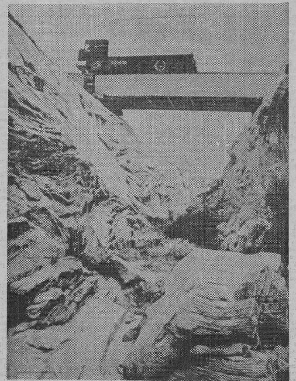
Aunque parezca increíble, el puente sobre el que pasa este camión es de cartón ondulado. — (Foto EFE).
