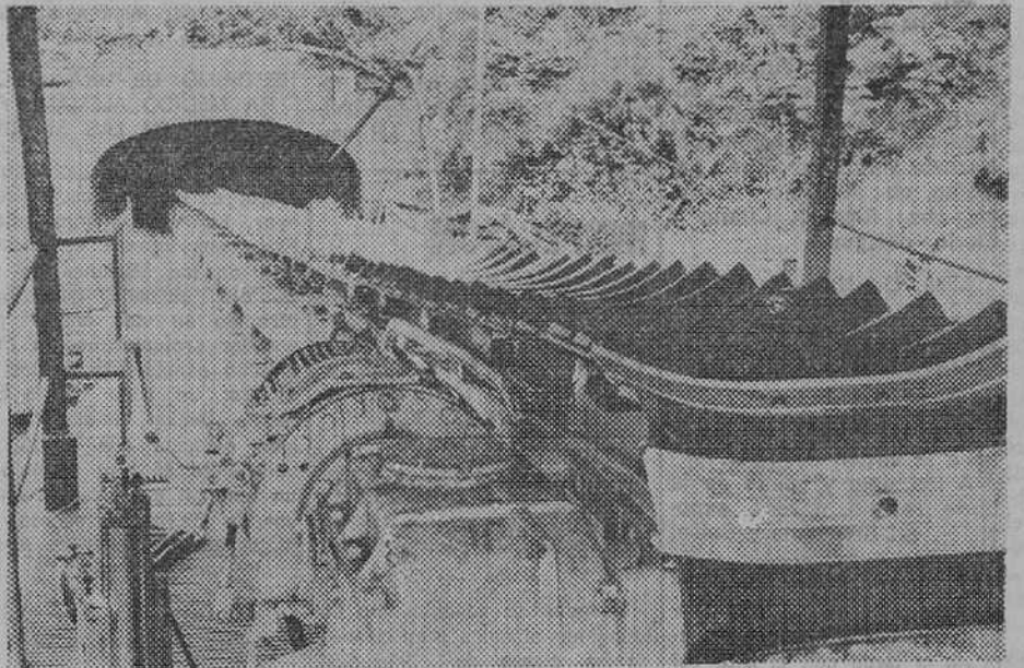
Hunosa (Hulleras del Norte, S. A.), la mayor empresa carbonífera de España, está dotando a las minas de hulla de la cuenca asturiana de los mejores elementos, como esta cinta transportadora, a base de aluminio y goma, para transporte del material y mineros, cinta que está considerada como la mayor de Europa. (Foto EFE-FIEL).
