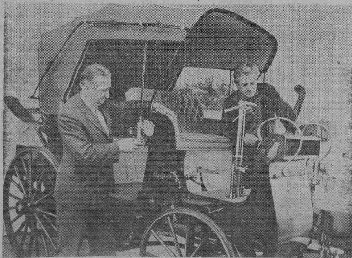
Se trata del "Präsident", el primer coche fabricado por la empresa Tatra de Miravia y que en 1897 dejó boquiabiertos a los habitantes de Praga. Ahora, la Tatra acaba de recuperar este su primer vehículo a motor, aunque se trata sólo de una copia perfecta, construida por un grupo de técnicos del Museo Técnico de Praga y del Museo del Automóvil de la Tatra. — (Foto FIEL-CTK).
