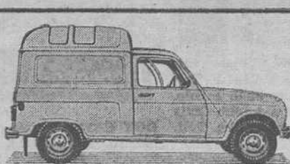
Sobreelevada Carga 425 kg. Altura útil 1,307 m. Volumen útil de carga 2,08 m 3
