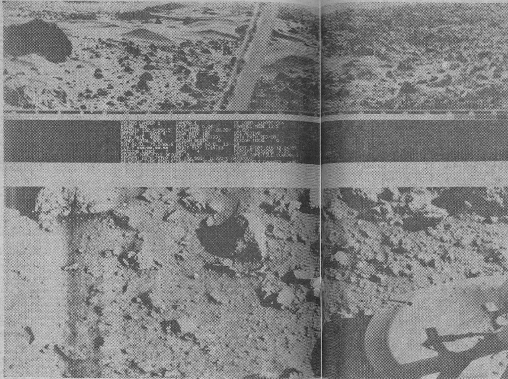
Dos vistas de la superficie del planeta Marte tomadas por la sonda Vikingo: en el "planeta rojo" se detecta una actividad química incomprensible por el momento. (Foto EFE-FIEL)
