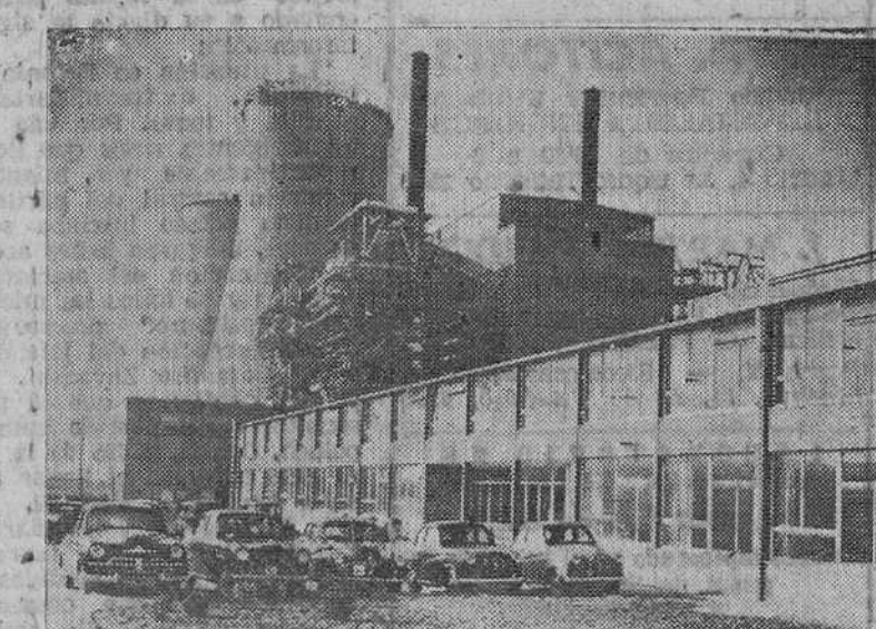
Vista parcial de la primera central electroatómica en gran escala del Mundo, construida en Calder Hall, Cumberland (Inglaterra). En primer término se ven las oficinas y al fondo, las torres de enfriamiento. — (Foto C.)
