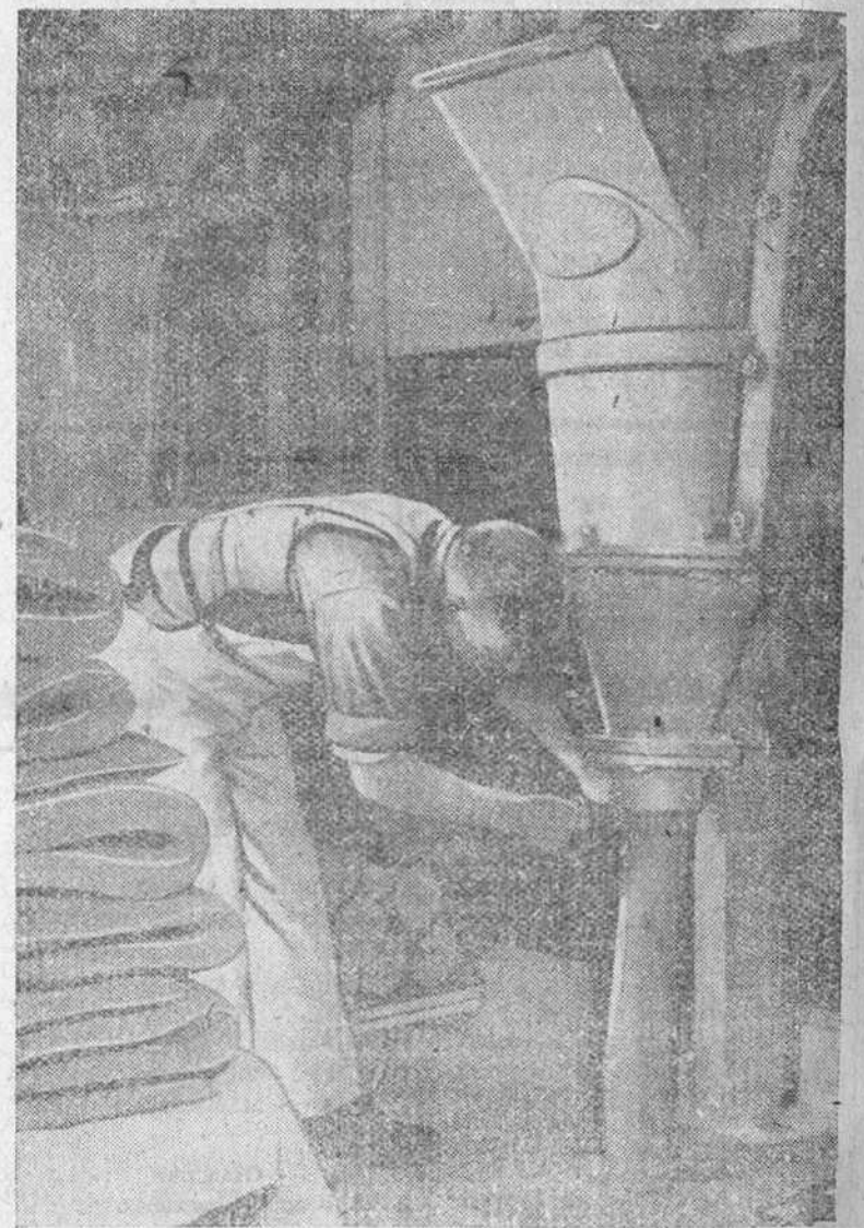
En una moderna fábrica de cerámica, en Gran Bretaña, este operario atiende al filtro-prensa por donde las tartas de arcilla pasan a la amasadora que mezcla el producto y le da homogeneidad hasta expulsarle por el grueso tubo que aparece en la parte inferior del grabado (Foto Calpe)
