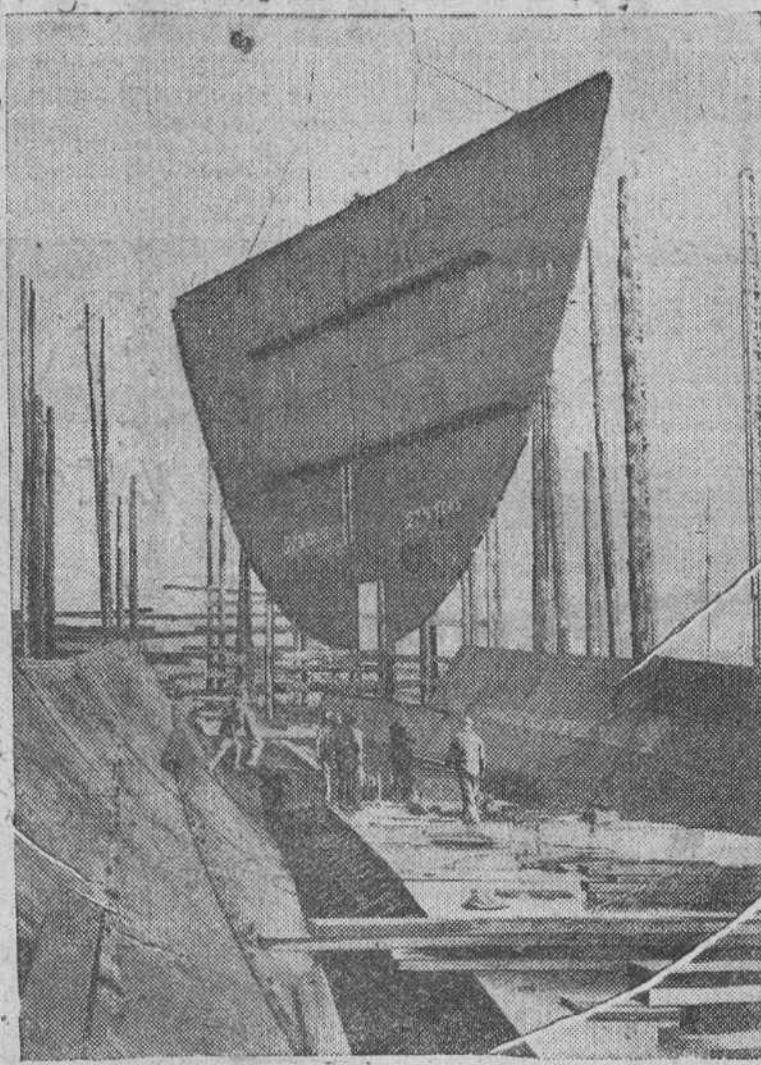
En el noticiero NO-DO que exhibieron ayer algunas de las pantallas de los cines locales se ofreció un reportaje sobre la construcción de buques prefabricados en Inglaterra. Esta foto que publicamos representa a unos obreros colocando una enorme pieza, que formará parte de la quilla de un buque de tonelaje medio. Con el nuevo método se ahorran más de 900 toneladas de acero en la construcción de buques de la clase "Orcada" y un aumento en su tonelaje. Con estas piezas prefabricadas se consigue además reducir la vibración y ahorra un 25 por ciento de tiempo en la construcción de unidades navales.—(Foto Calpe)
