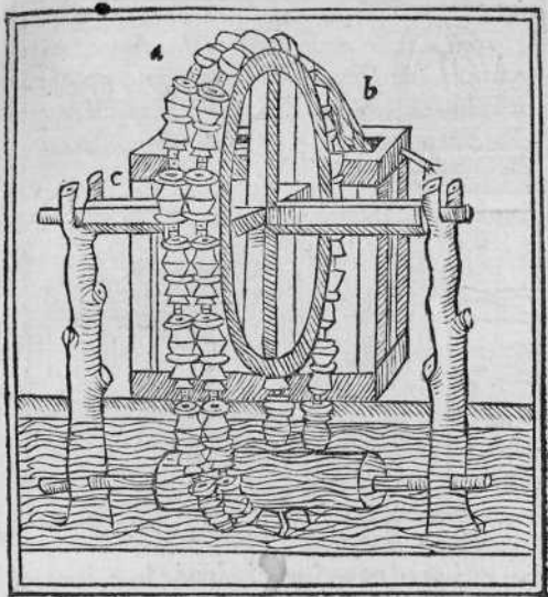
a. fituli- b. castel- lum. c. axis.
