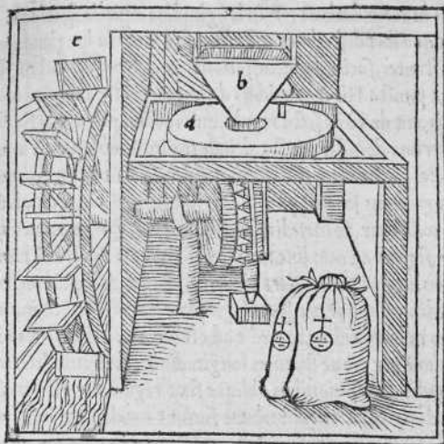
a. mola. b. infu- dibulum c. pinna rota.
