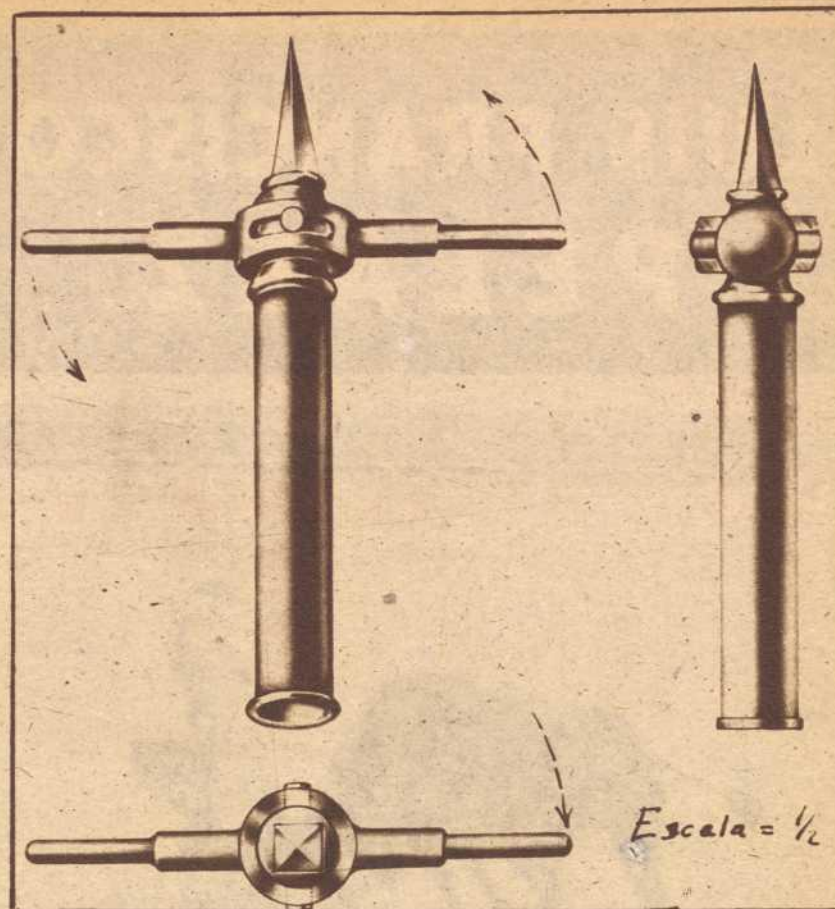
Croquis de la puya propuesta por don Manuel Pérez Candela
