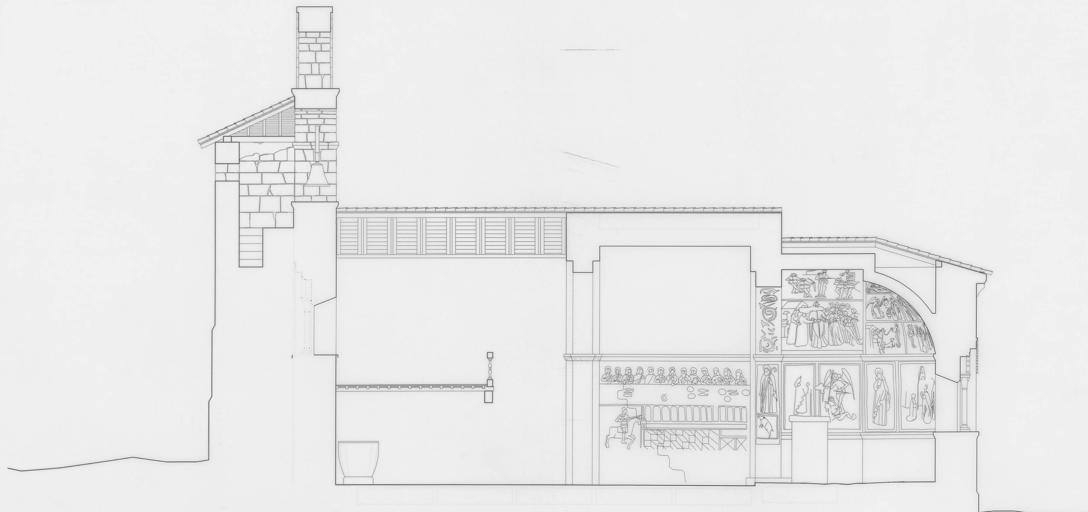
SECCION LONGITUDINAL
