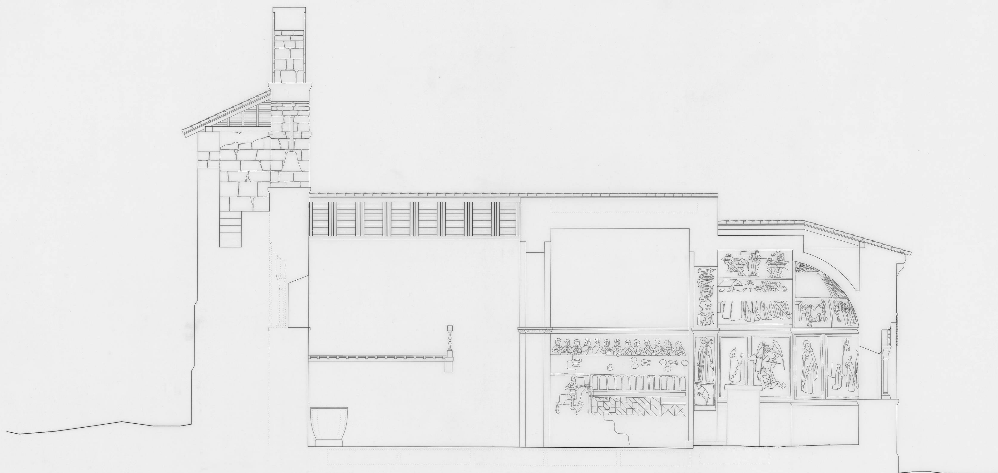
SECCION LONGITUDINAL
