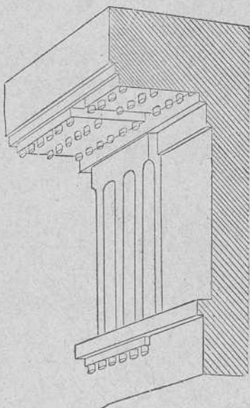
FIG. 10. — DÉTAIL DES MUTULES.
