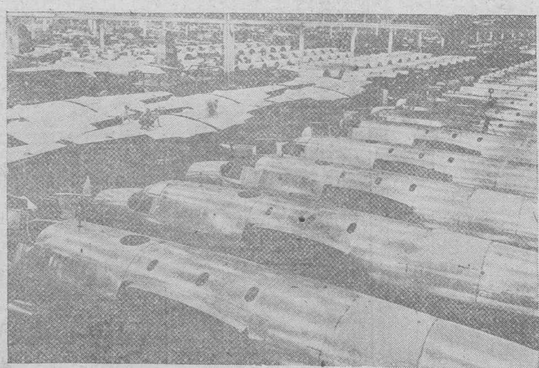
El taller de montaje final de la fábrica de Glenn L. Martin, en el Este de los Estados Unidos, donde se produce el bombardero B-26. Tiene dos motores de 1.850 c.v. cada uno y hélices de cuatro palas, que le desplazan a una velocidad superior a 450 kilómetros por hora
