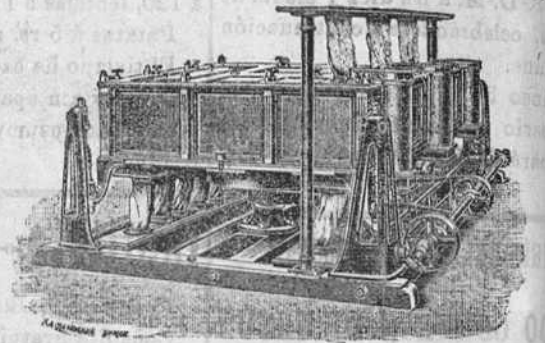
PLANSICHTER (último modelo).—Construcción Daverio
