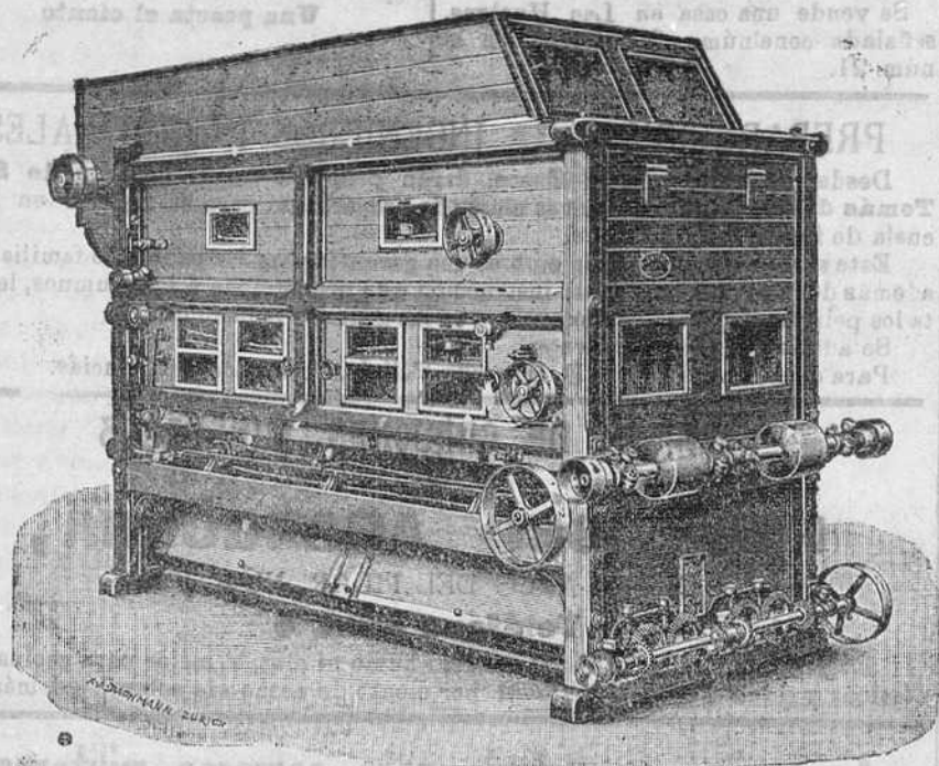
COLUMNA DESPUNTADORA
