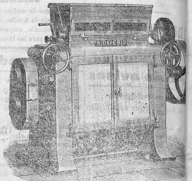
PLANSICHTER (último modelo).—Construcción Daverio
