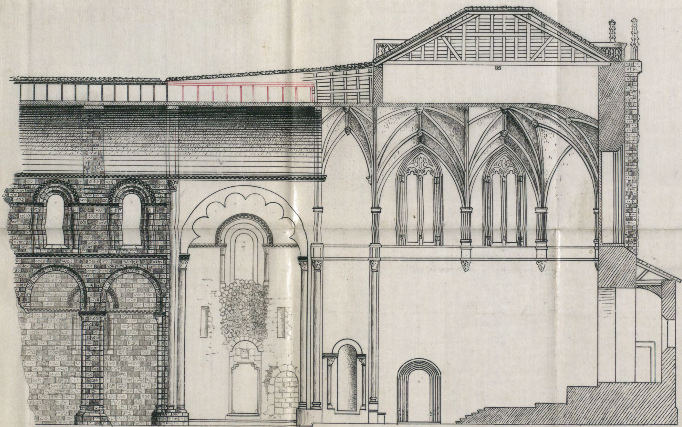
Sección Longitudinal
