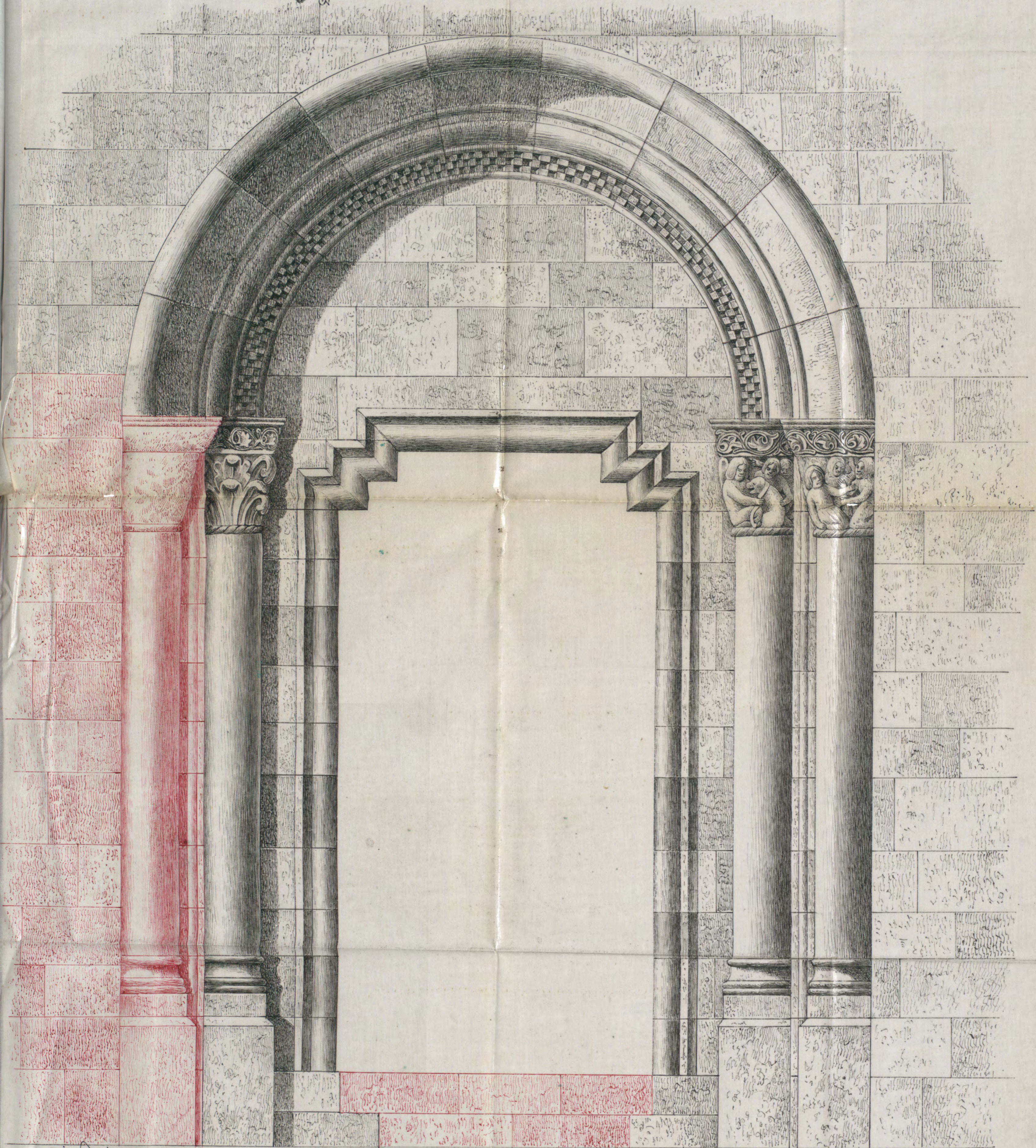
Puerta Norte del crucero - Detalle
