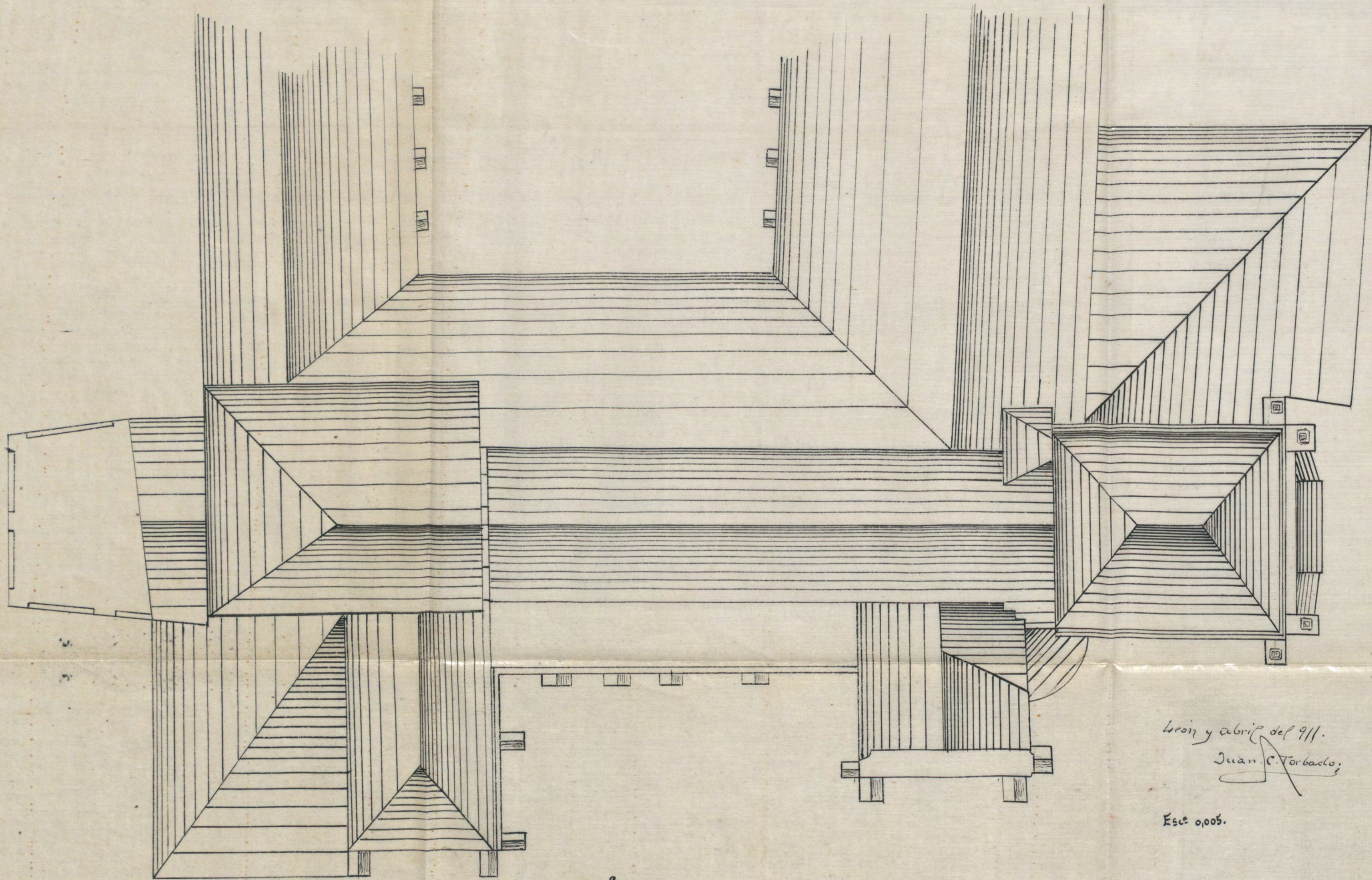
Planta de cubiertas
