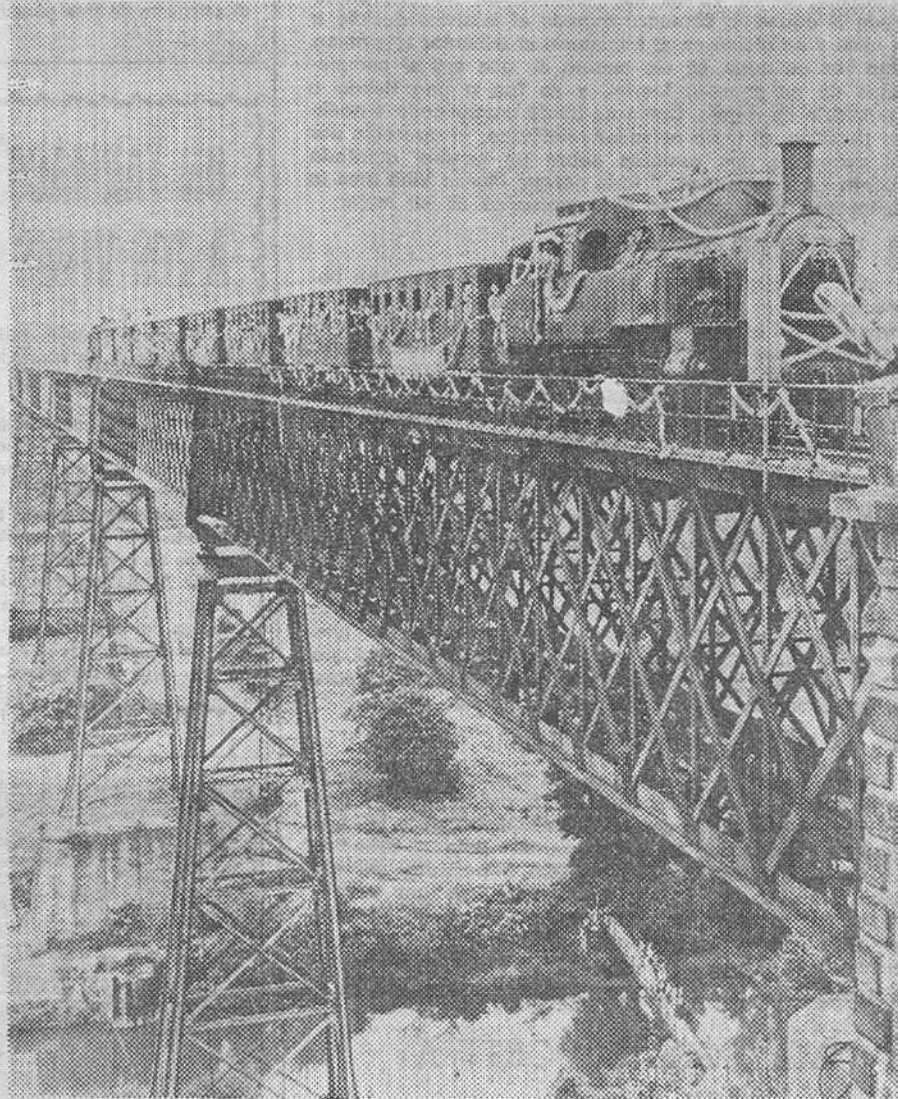
Se trata del viaducto para trenes sobre el río Jihlava, en Checoslovaquia, de 373,5 metros de largo y 1.500 toneladas de peso. Muy pronto será sustituido por otra construcción. Empero, debido a su estructura y su interés para ingenieros y estudiantes técnicos, el viejo puente, construido hace 108 años, será incorporado al Museo Técnico de Brno. — (Foto FIEL-CTK).
