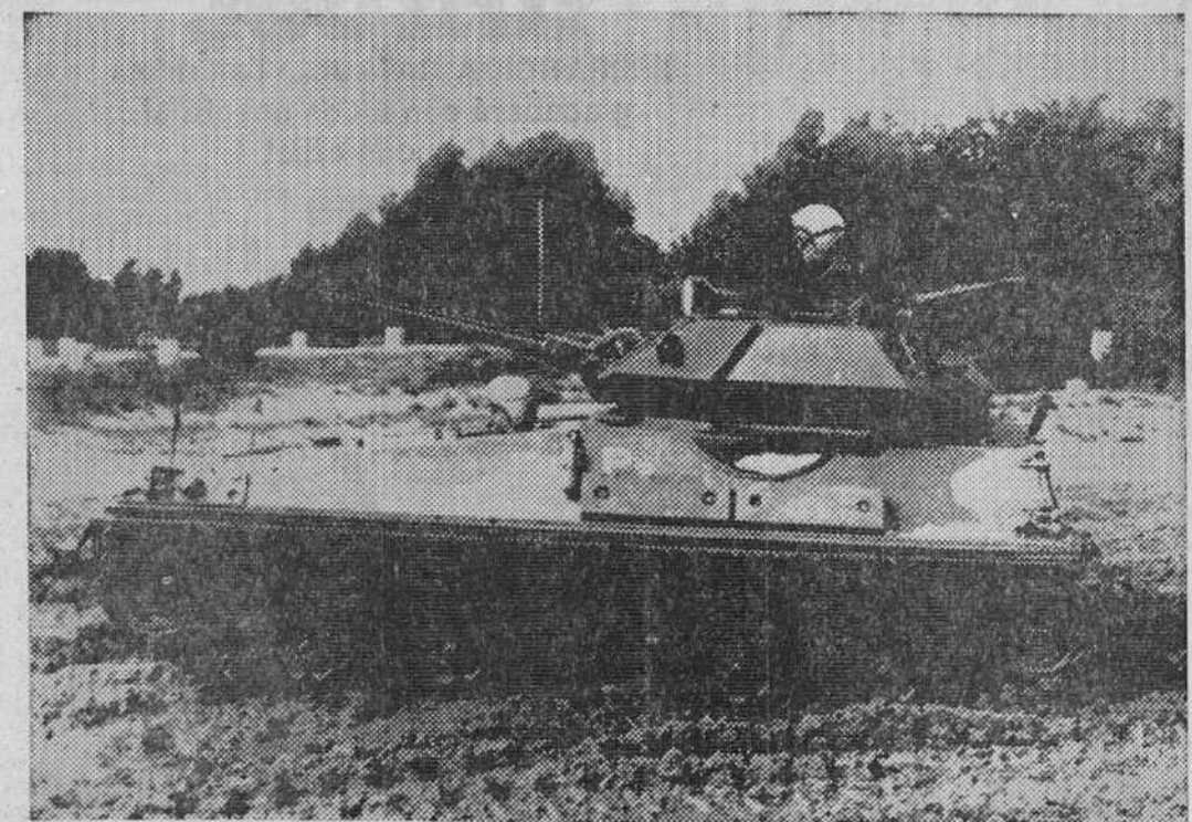
Este es el prototipo de pruebas de un nuevo tanque británico que actualmente es perfeccionado por el Ministerio de Defensa y la Alvis Ltd. Se denomina «Scorpion» y es el primer vehículo blindado del mundo construido casi totalmente de aluminio. Pesa ocho toneladas y ha sido ideado para ser utilizado en condiciones que exijan elevada relación peso-fuerza. Es muy adecuado para operaciones en terrenos pantanosos o cubiertos de nieve, donde vehículos más pesados se atascarian. Otras de sus ventajas es que es transportable por vía aérea. Lleva un motor ordinario Jaguar XK exalíndrico de 4.200 c. c. — (Foto FIEL).
