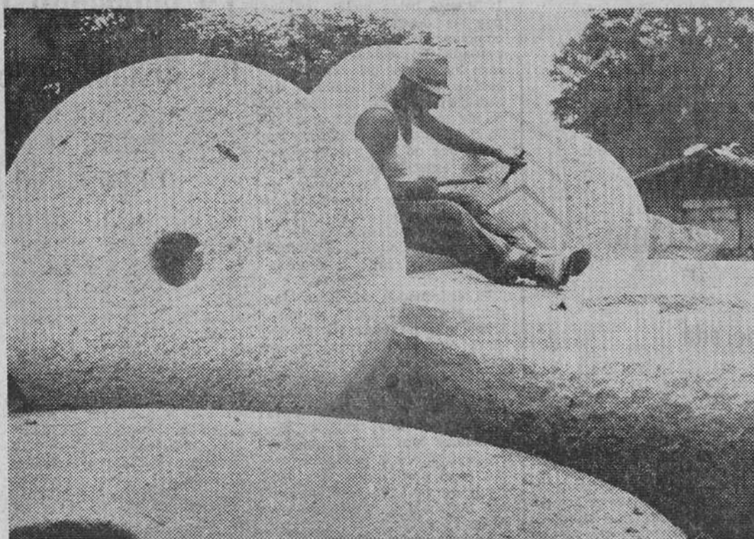
En los tiempos de las modernas trituradoras y prensas hidráulicas, todavía se siguen utilizando estos enormes bloques cilíndricos de granito, para moler la aceituna en algunos lugares de Italia. Este picapedrero realiza, a golpe de martillo, las estrías de las ruedas, en un lugar cercano al Lago Maggiore, en Bavona. Su tarea es tan delicada como la de un escultor (Foto FIEL)
