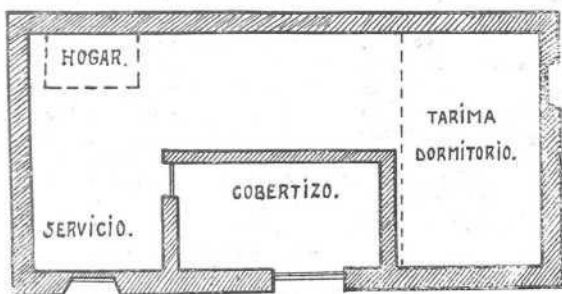
PLANTA Y ALZADA DEL REFUGIO DEL CLUB ALPINO ESPAÑOL
