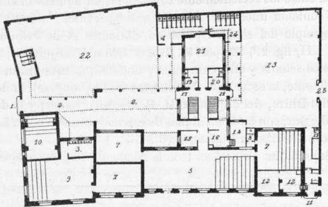
Planta baja.
