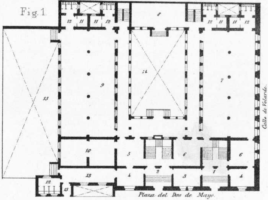
Planta principal.
