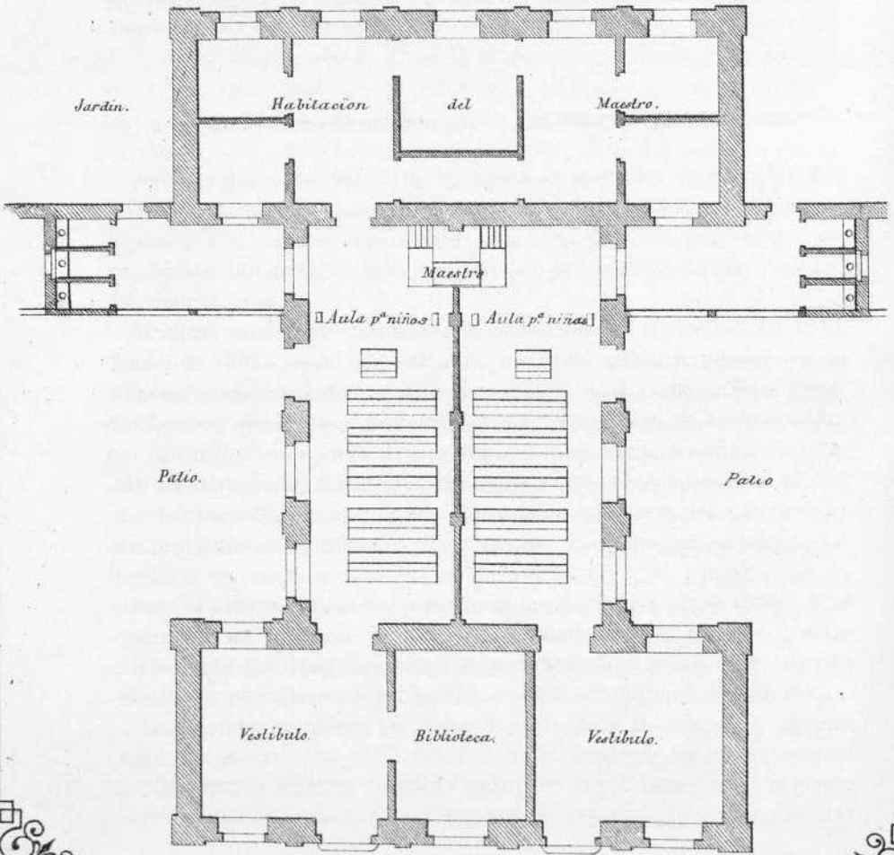
Planta
