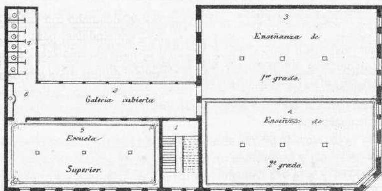
Planta del 2.º piso.
