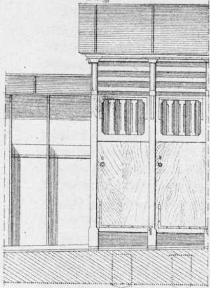
Alzado. Fig. 1.
