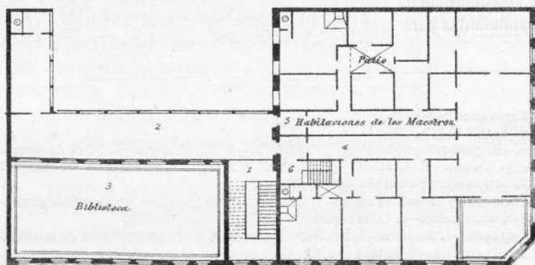
Planta del 2.º piso.
