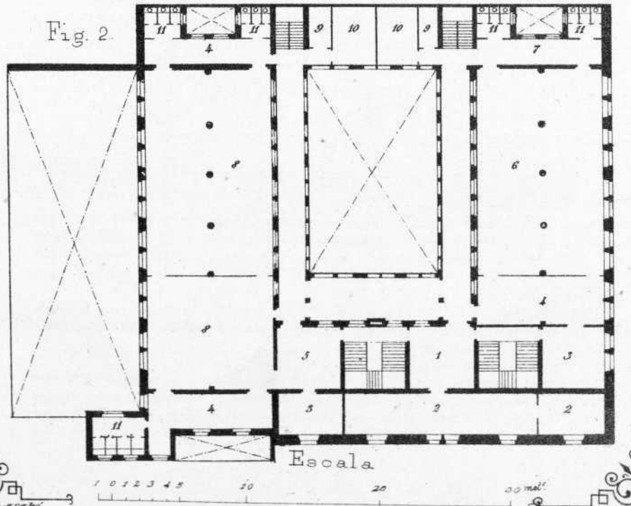
Planta principal.
