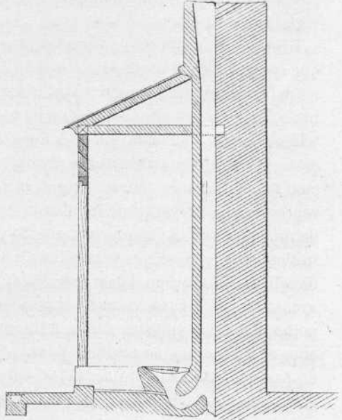
Seccion. Fig. 2.
