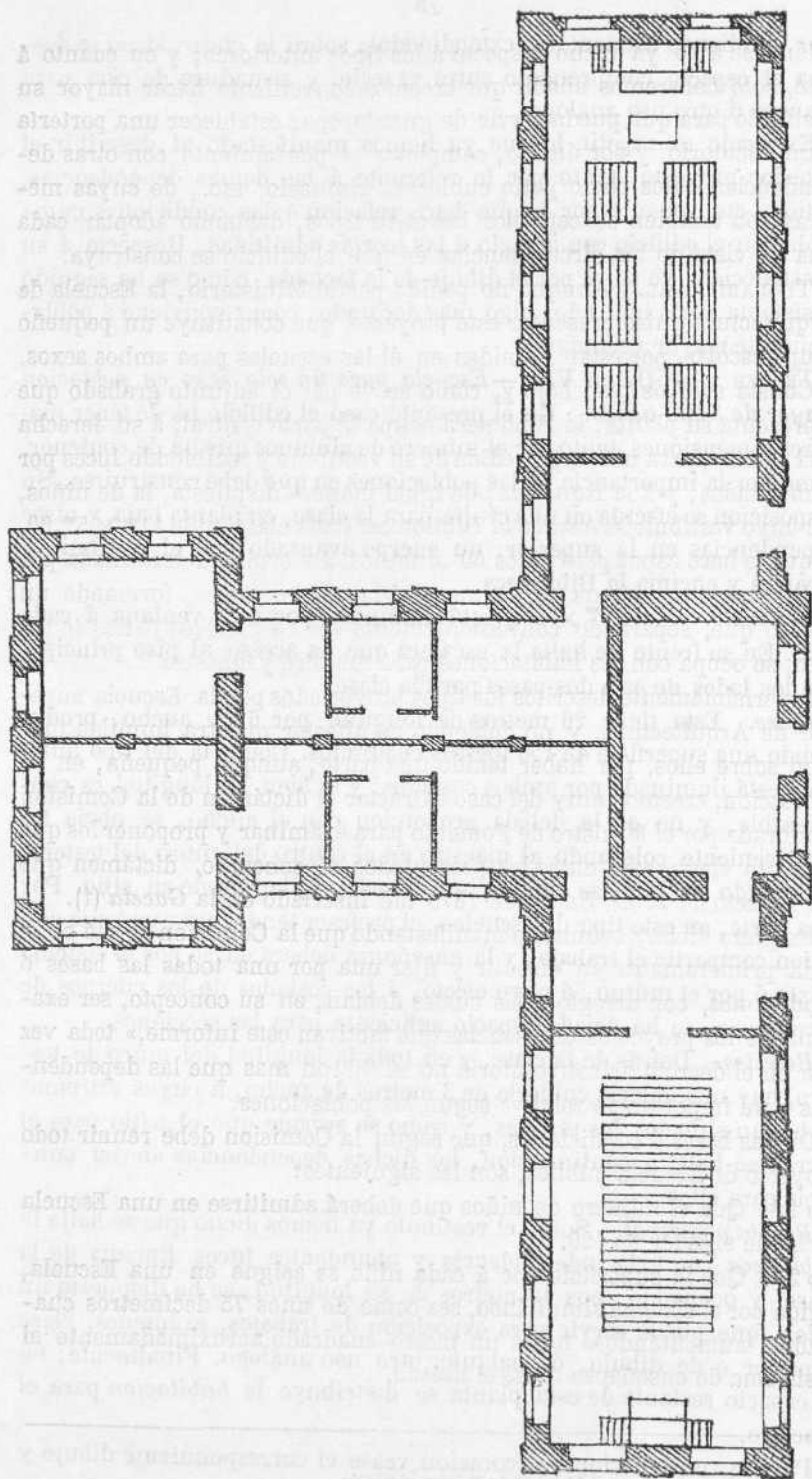
Tipo adicional de la Escuela de Arquitectura. — Escala de 0 m ,005 por metro.
