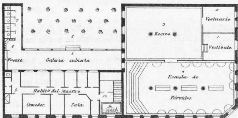
Planta del 1.º piso.
